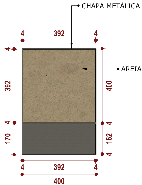
01 VISTA SUPERIOR ESCALA: 1/10 - CAIXA DESMUNICIAMENTO
