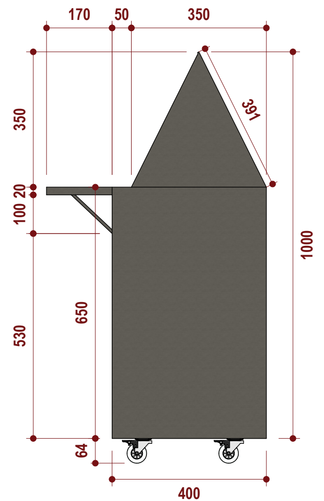
04 VISTA LATERAL ESCALA: 1/10 - CAIXA DESMUNICIAMENTO
