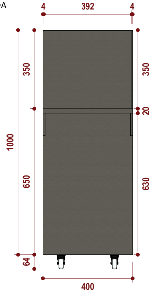
03 VISTA FRONTAL ESCALA: 1/10 - CAIXA DESMUNICIAMENTO
