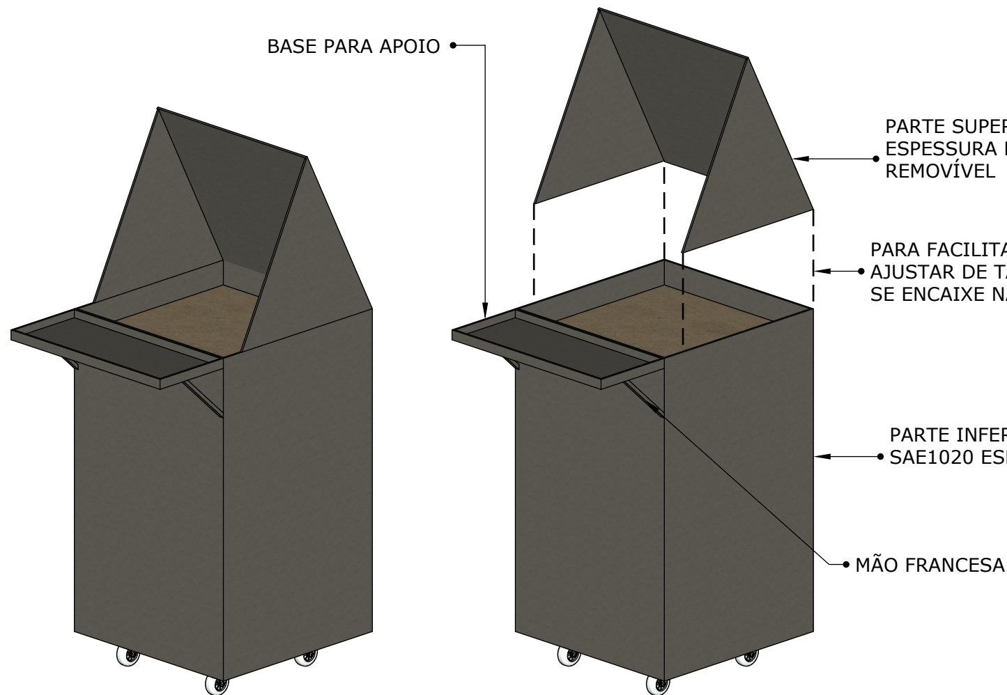
05 VISTAS ISOMÉTRICAS ESCALA: 1/10 - CAIXA DESMUNICIAMENTO
