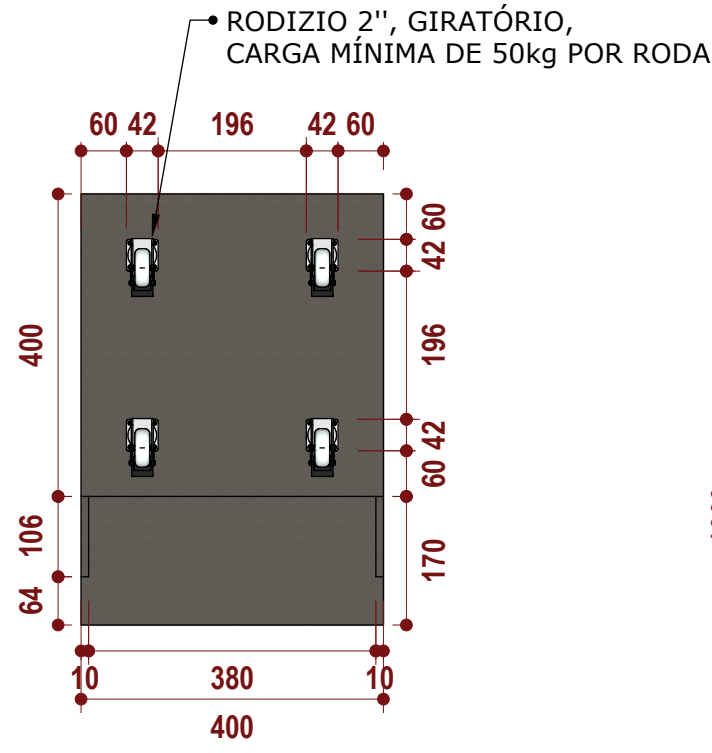
02 VISTA INFERIOR ESCALA: 1/10 - CAIXA DESMUNICIAMENTO
