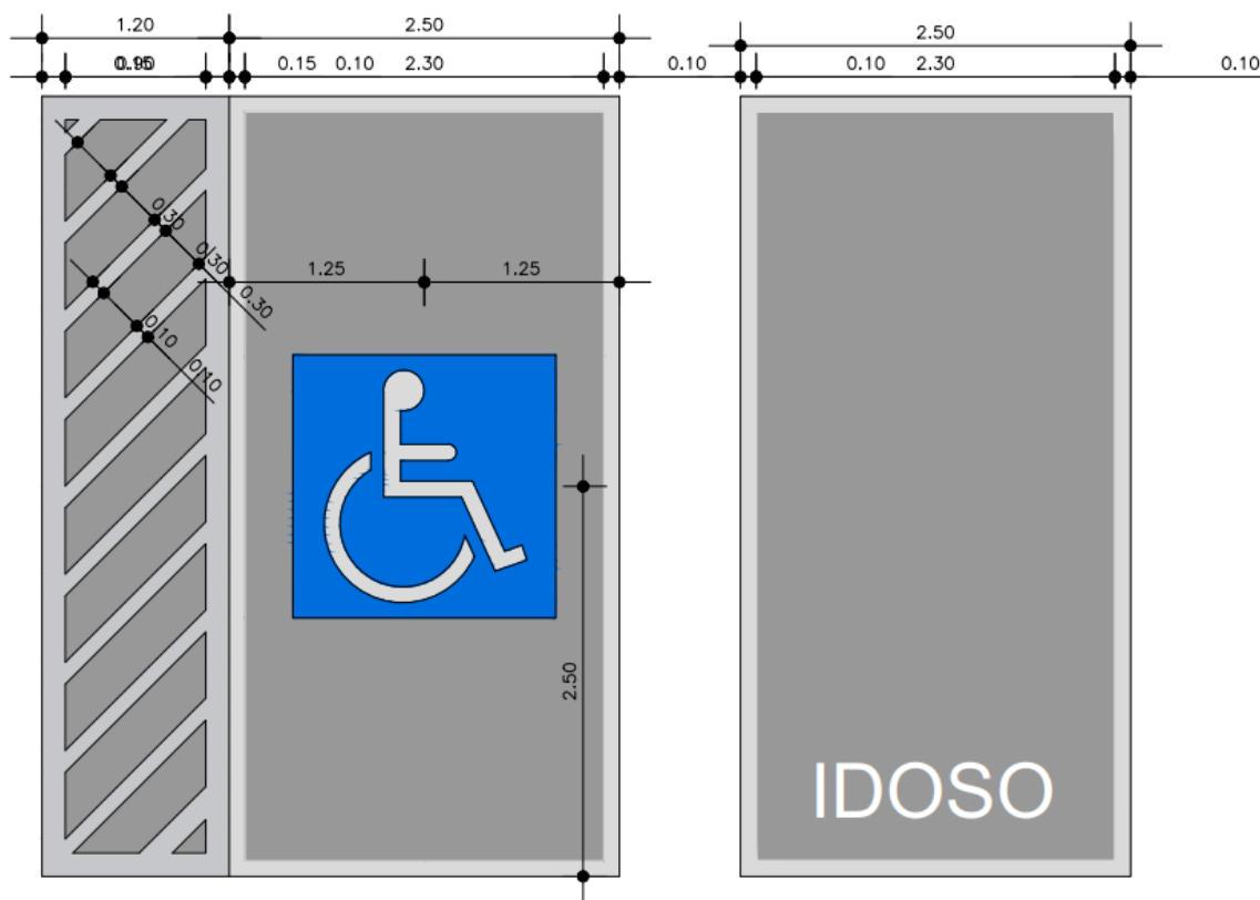
MARCAÇÃO DE PINTURA NO PISO DE ESTACIONAMENTO
