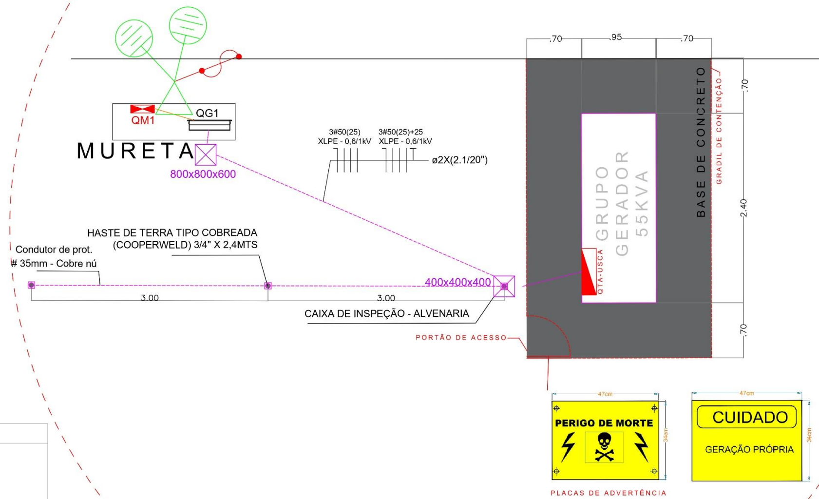
PLANTA GRUPO GERADOR CARENADO
