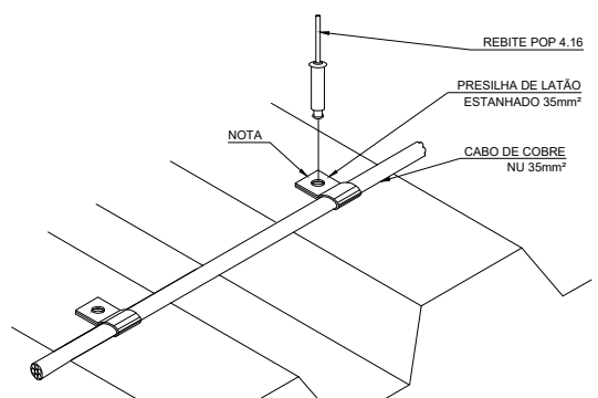
PRESLIHA DE FIXAÇÃO EM TELHA METÁLICA DETALHE 08
