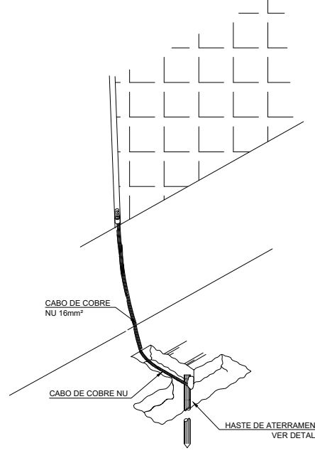
INTERLIGAÇÃO DA MALHA DE ATERRAMENTO COM ALAMBRADO, BASE DE POSTE E CORRIMÃO DETALHE 15
