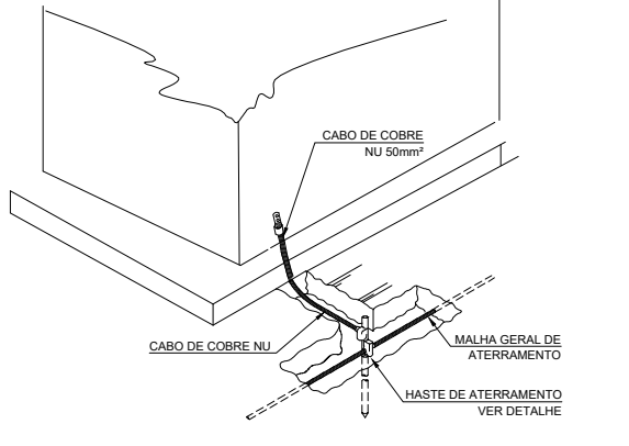
INTERLIGAÇÃO DA MALHA DE ATERRAMENTO COM CABO E COBRE NA ESTRUTURA
