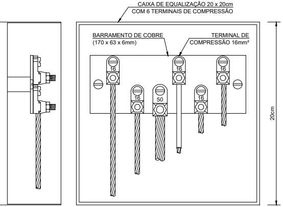
CAIXA DE EQUALIZAÇÃO DOS POTENCIAIS 20 x 20cm DETALHE 11
