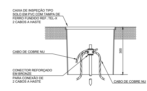
DETALHE DE CONEXÃO E SOLDA DA HASTE DE ATERRAMENTO DETALHE 16
