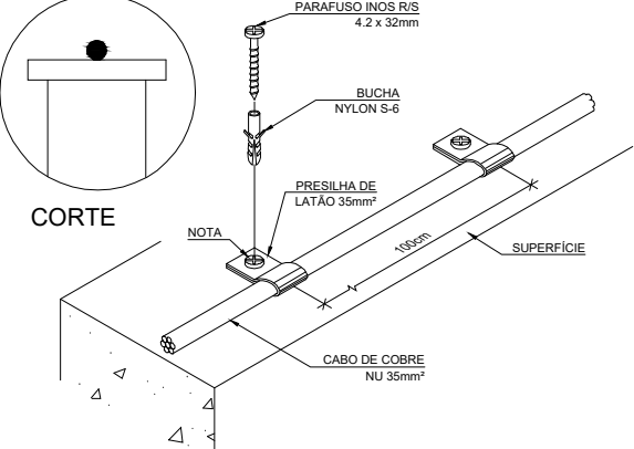
FIXAÇÃO GERAL DE CABO DE COBRE DETALHE 13
