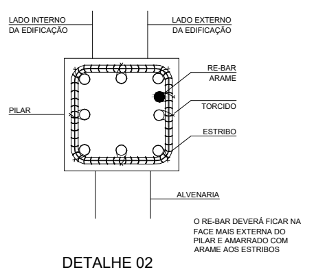
DETALHE 02
