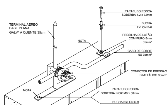
TERMINAL AÉREO CAPTOR BASE HORIZONTAL 35cm E CABO DE COBRE FIXADOS EM ALVENARIA DETALHE 09
