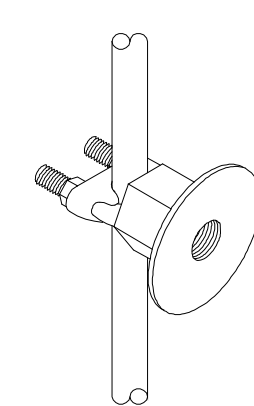
CONECTOR ATERRINSERT COM DISCO EM LATÃO DETALHE 12
