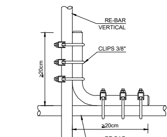
DETALHE 07
