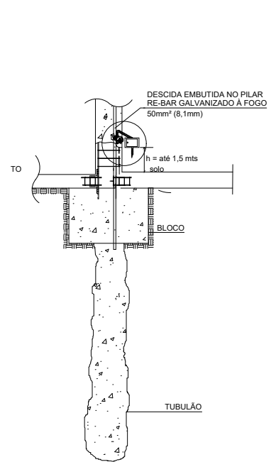
ATERRAMENTO NA FUNDAÇÃO TUBULÃO SIMPLES E BALDRAME DETALHE 04
