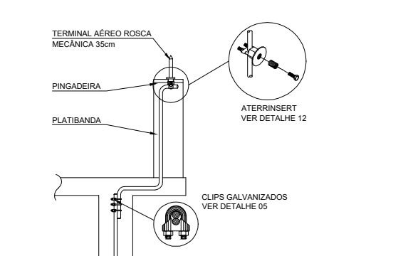
INTERLIGAÇÃO DO RE-BAR DE DESCIDA COM O TERMINAL AÉREO ROSCA SOBERBA DETALHE 10
