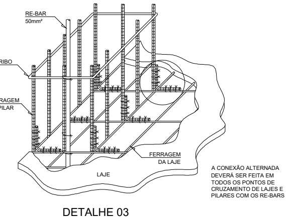
DETALHE 03
