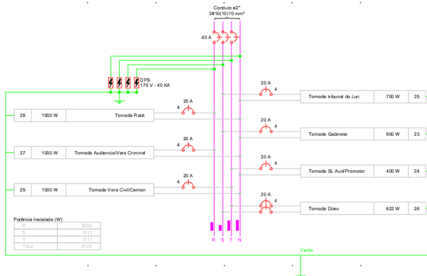
QD2 (QUADRO LUZ E TOMADAS)
