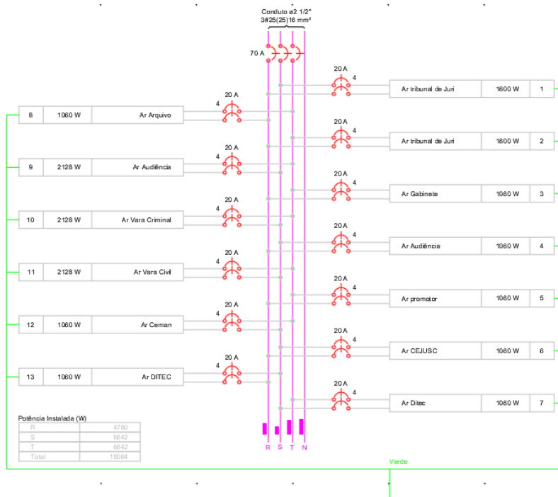
QD3 (QUADRO AR CONDICIONADO)
