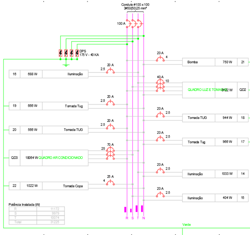
Diagrama multifilar do Quadro QD1:
