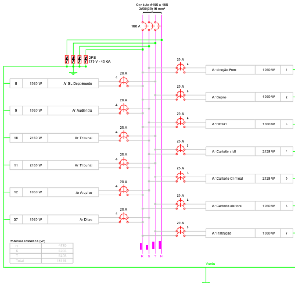
QD2 (QUADRO AR COND)
