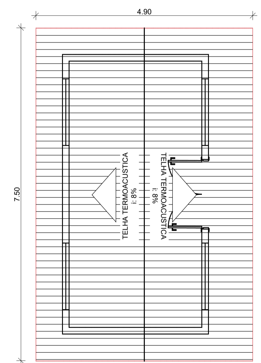
PLANTA DE COBERTURA Esc. 1/50
