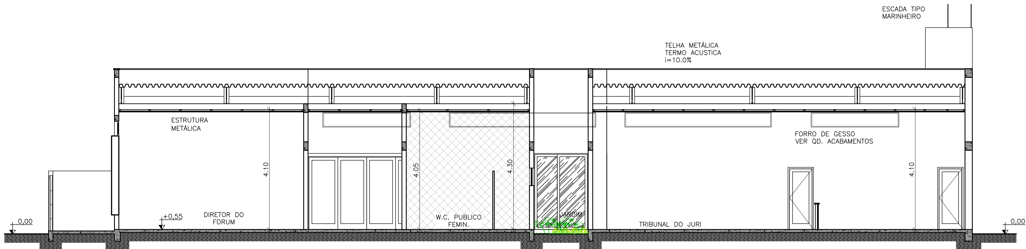
CORTE CC Esc. 1/75
