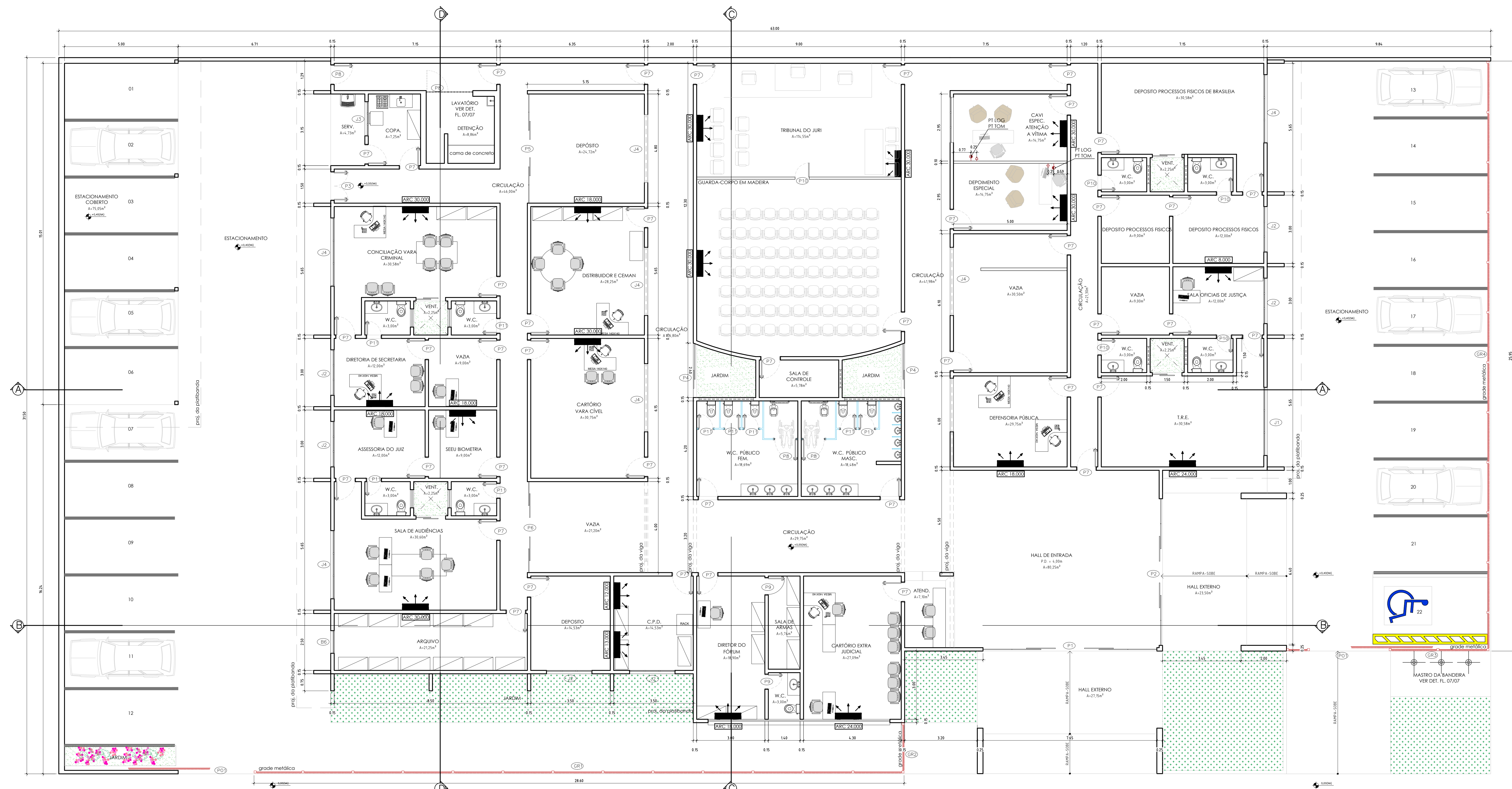
PLANTA BAIXA / LAYOUT Esc. 1/75
