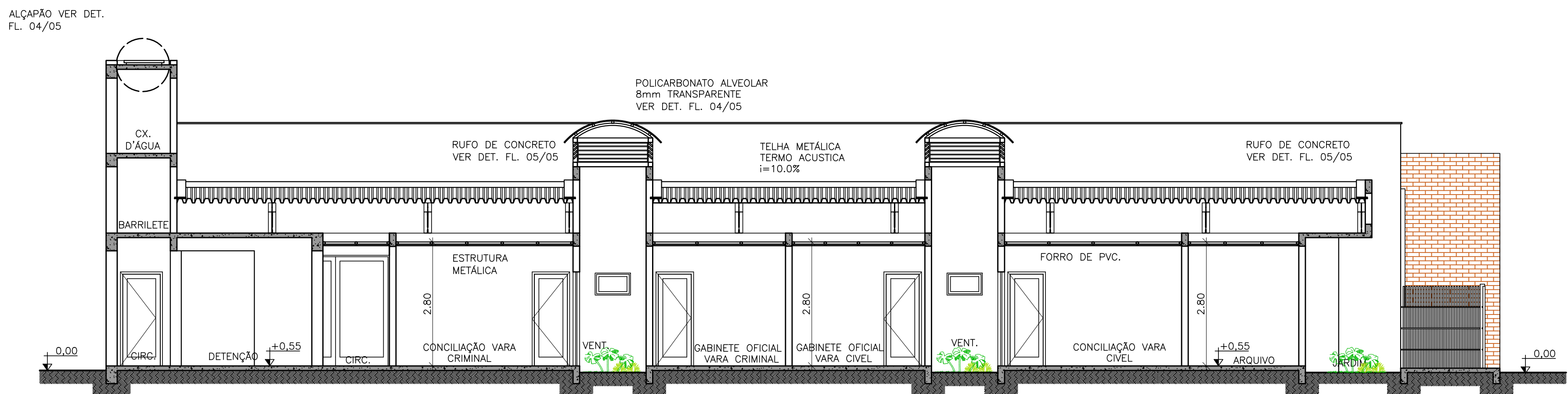
CORTE DD Esc. 1/75
