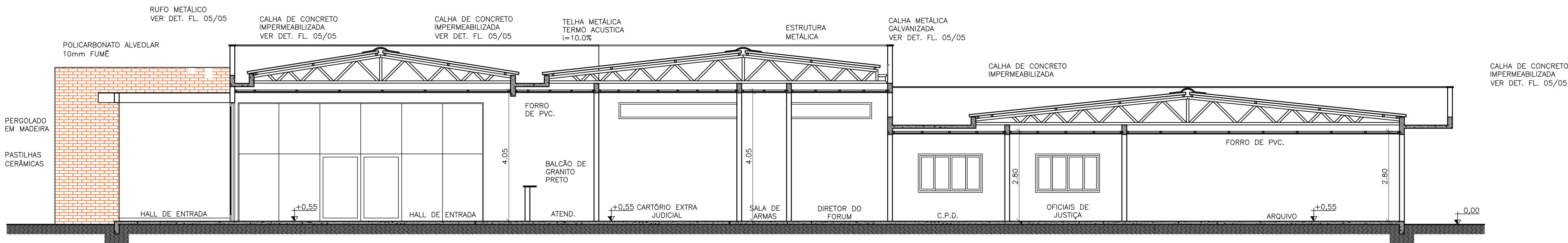
CORTE BB Esc. 1/75
