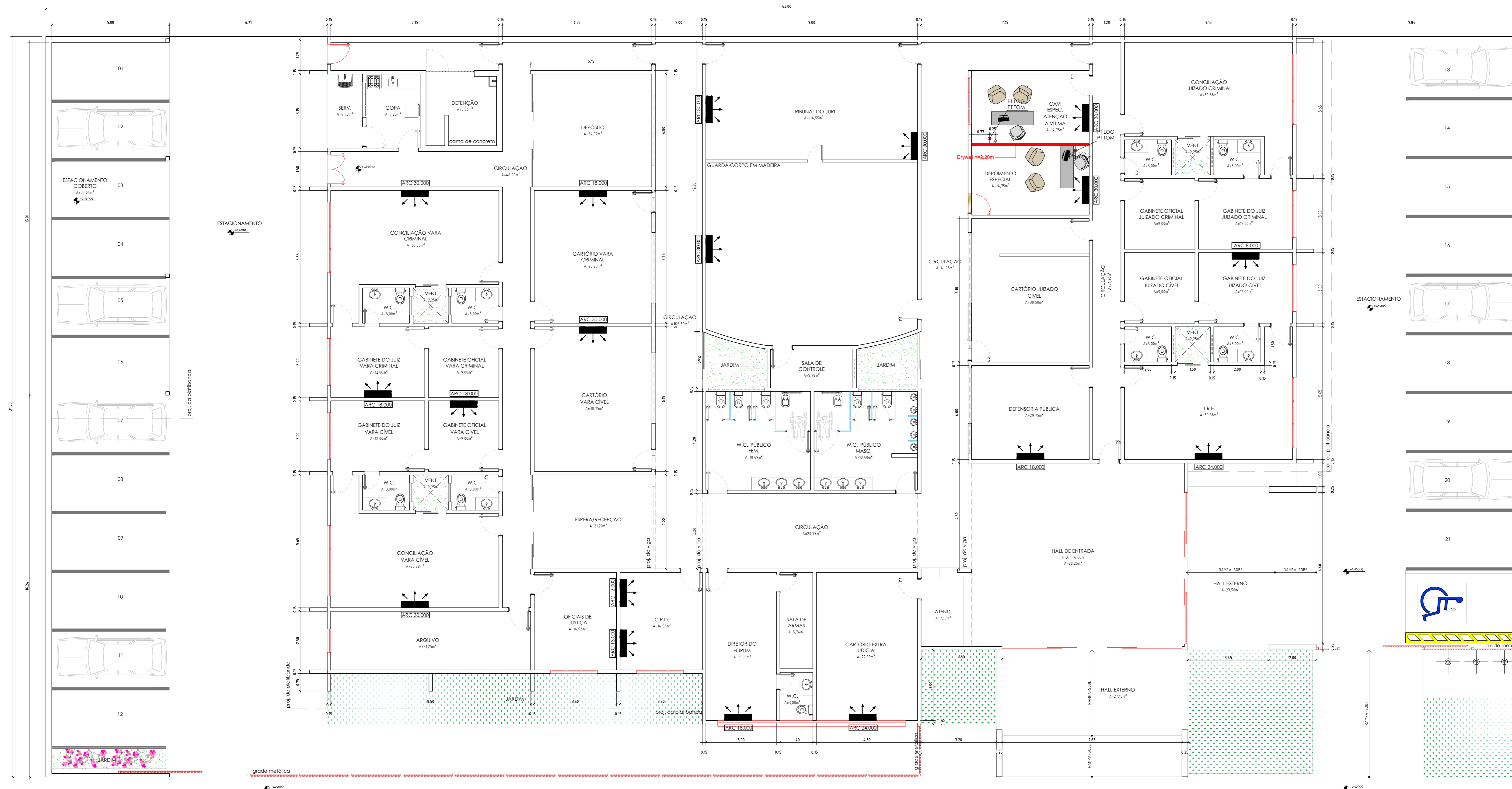
PLANTA BAIXA - REFORMA E ADEQUAÇÃO Esc. 1/75
