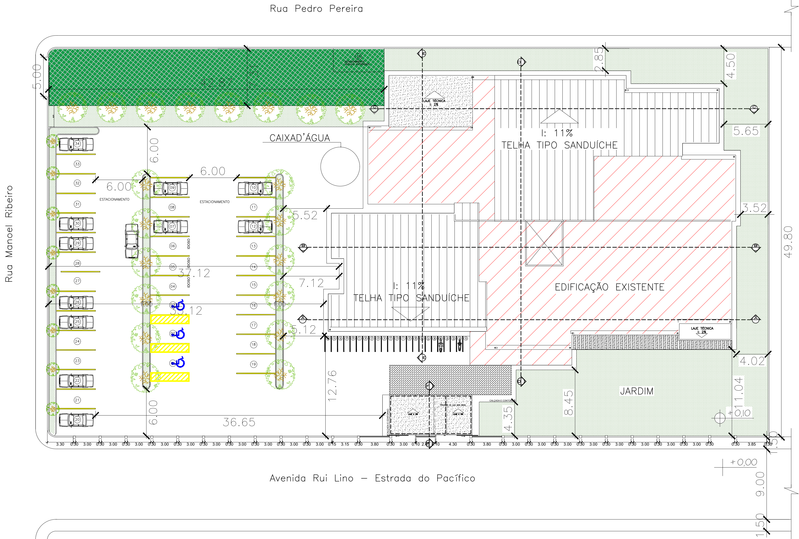
PLANTA DE COBERTURA E IMPLANTAÇÃO - 2ª ETAPA ESC.: 1/200
