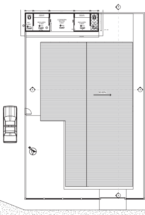
3 COBERTURA 1 : 100
