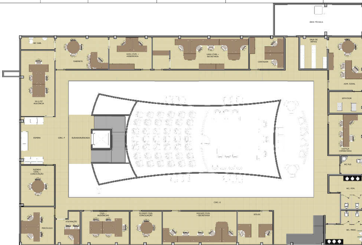
1 LAYOUT - PAV. SUPERIOR 1:50
