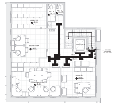
2 PLANTA BAIXA. PAV. SUPERIOR ESCALA: 1 : 75
