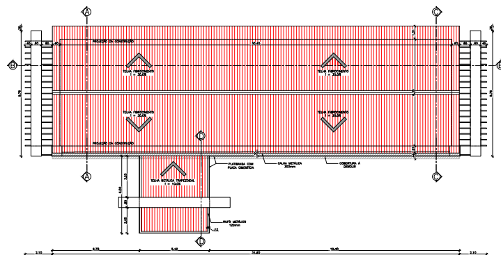
PLANTA DE COBERTURA - CIC de PORTO ACRE REFORMA & AMPLIAÇÃO - 2015
